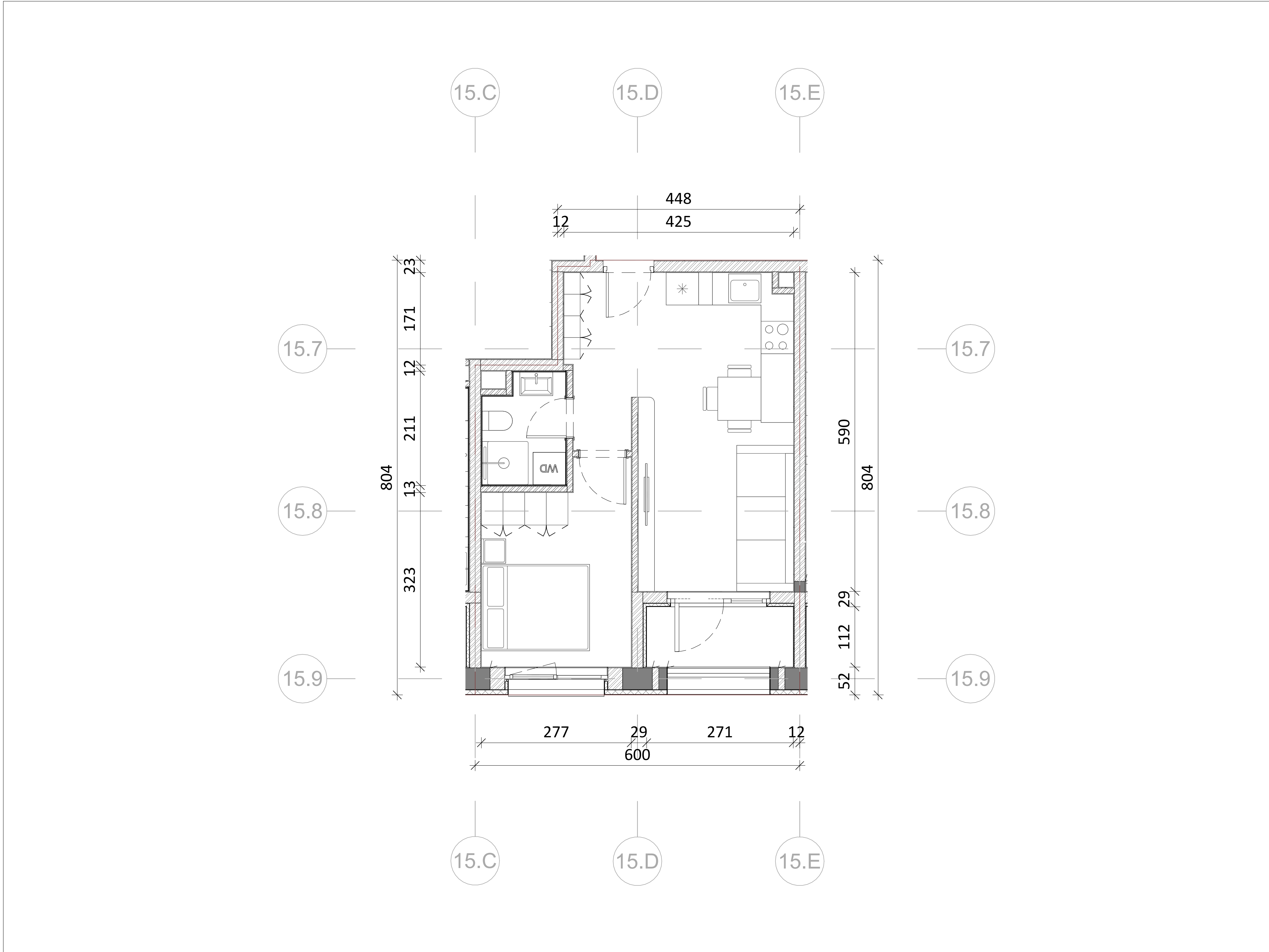
VENDNDODHJA E APARTAMENTIT NE PLANIN E KATIT TE PARE SH. 1:1250
